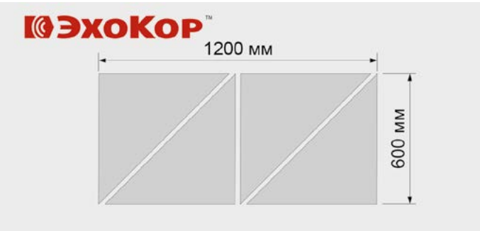
Вариант комплекта треугольников ЭхоКор Т 50
